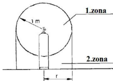
3.2. att. Sprādzienbīstamais zonējums ap gāzes balonu
