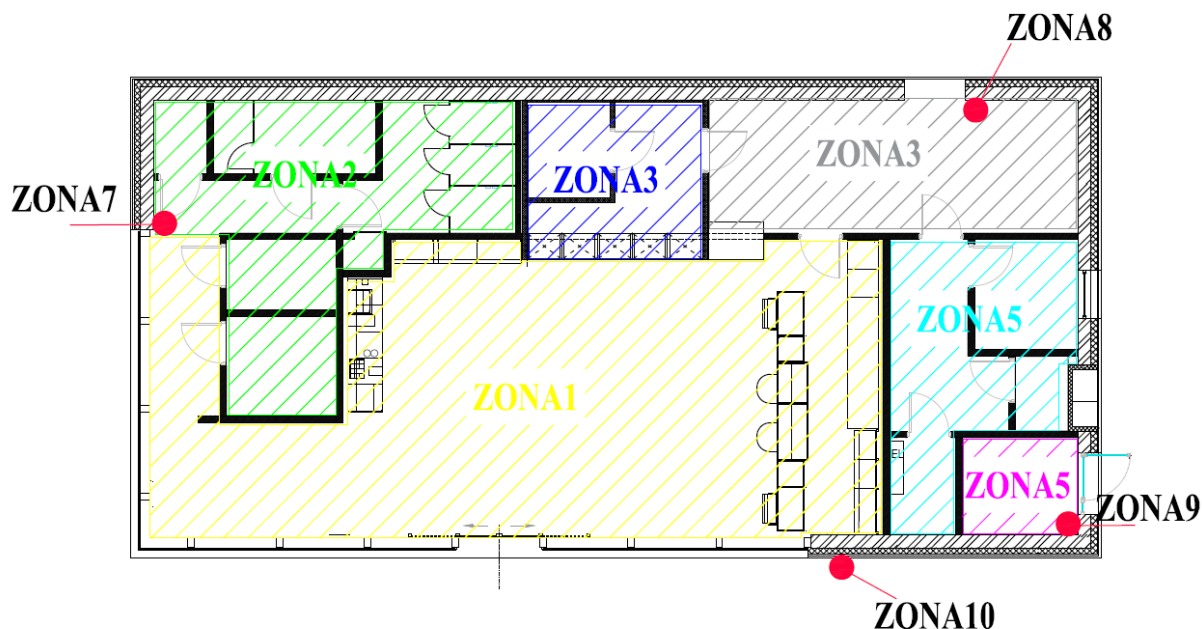
13.1. att. Uguns aizsargāto zonu sadalījums DUS "Bergī" degvielas uzpildes stacijas ēkā
