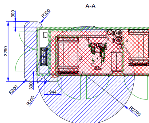
3.3. att. Sprādzienbīstamais zonējums kompresora stacijā un ap to (skats no augšas)
