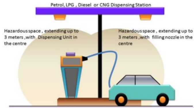
3.4. att. Sprādzienbīstamais zonējums automašīnas uzpildes laikā
